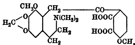
Narceine.
